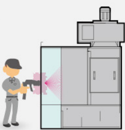
◎ 囲い式フード 制御風速 0.4m/sec
