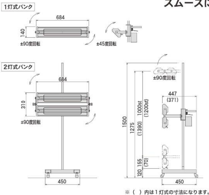
1・2 灯式ヒーター寸法図
