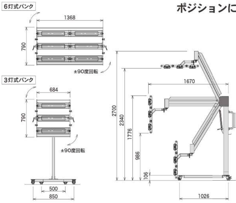
3・6 灯式ヒーター寸法図
